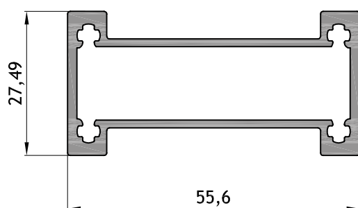
BA - 043 Parante Peso: 0,858 kg/m Largo: 6150 mm
