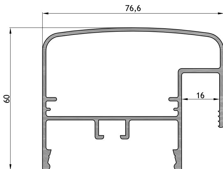
BA - 513 Pasamanos recto Peso: 1,363 kg/m Largo: 6150 mm
