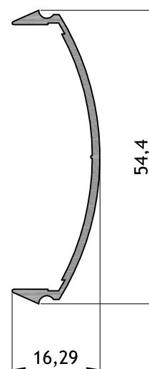
BA - 503 Tapa inferior pasamanos Peso: 0,266 kg/m Largo: 6150 mm
